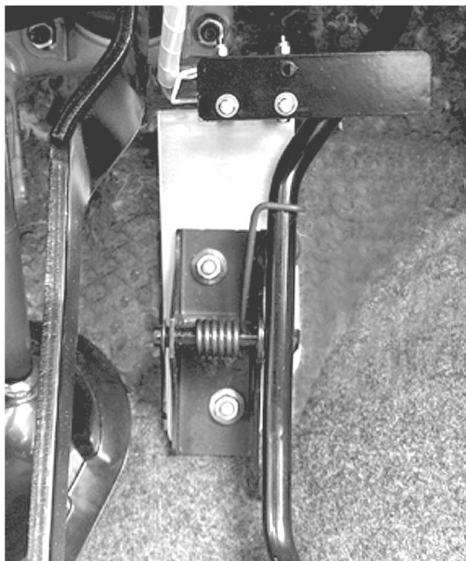
車両のアクセルリンケージとボディー の間にSDASを取り付けます
