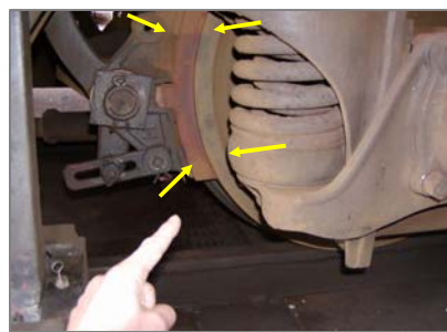
鉄道車両ブレーキ位置
